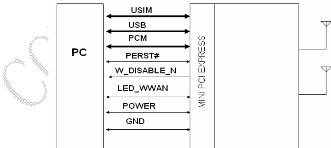
Figure 1-3 Mini PCI Express identification
